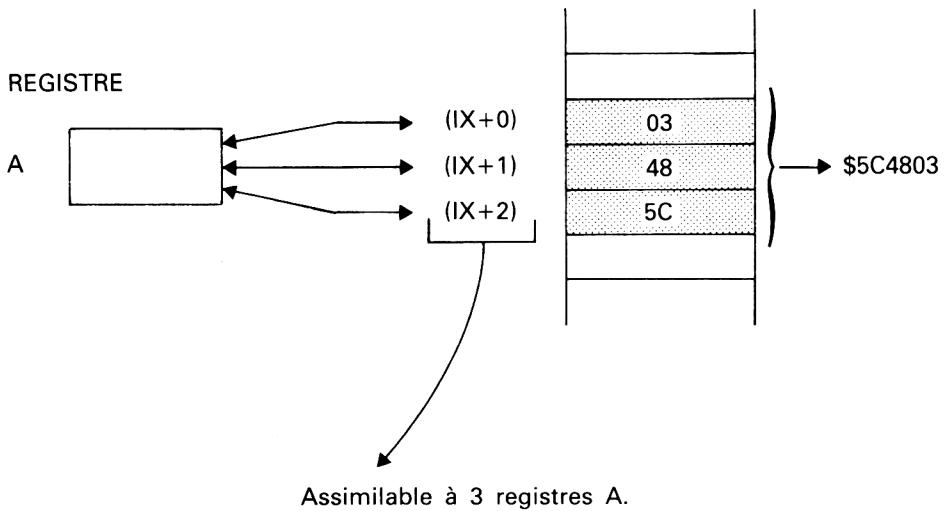
Accumulateur 24 bits.
